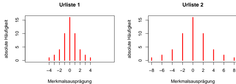
Stabdiagramme zu Urlisten mit identischem Mittelwert, Modus, Median
